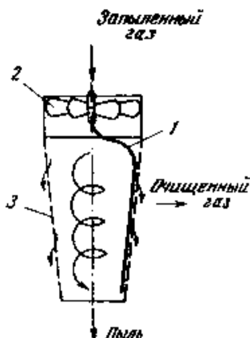
Рис. 1. Фильтровальный элемент проточного фильтра
