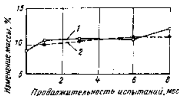
Зависимость изменения массы образцов асбестоцемента от продолжительности испытаний
