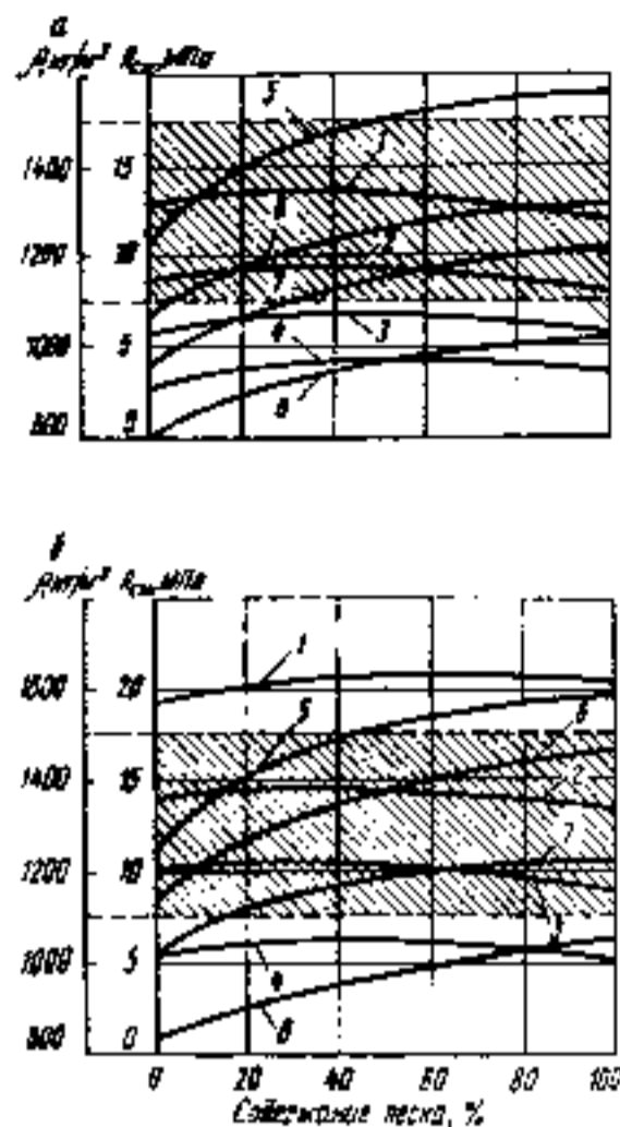
Рис. 2. Влияние расхода песка и опилков на прочность и среднюю плотность бетонов на основе гипсового вяжущего марок Г-5 (а) ГППСФ «Гипс» и ГП-7 (б) 1—8 — то же, что и на рис. 1.
