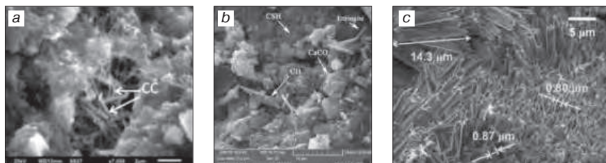
Рис. 8. Игольчатые кристаллы арагонита и их сростки, образовавшиеся под действием бактерий (слева направо): а – Bacillus sp . [9]; б – Bacillus subtilis [45]; с – Bacillus cohnii [35]
