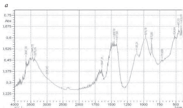
Рис. 3. ИК-спектры композиционного вяжущего без (а) и с ультрадисперсной добавкой (б)
