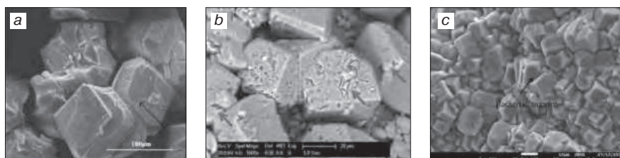
Рис. 7. Морфология псевдокубических сростков кристаллов кальцита, сформированных под действием бактерий: а – Bacillus sphaericus [37]; б – Bacillus sp [44]; с – Bacillus sphaericus [49]
