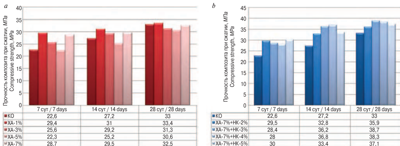
Рис. 9. Изменение прочности при сжатии R_{сж} силикатного композита в процессе твердения с добавлением хризотилового суспензии: а – без азотнокислого кальция; б – с использованием раствора азотнокислого кальция разной концентрации
