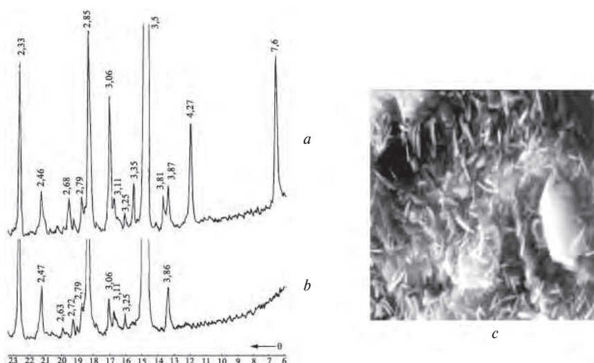
Рис. 7. Рентгенограмма гипсокерамического материала после обжига ( a ), выдержанного в воде ( b ) и его микроструктура ( c ) после хранения в воде (3000×)
