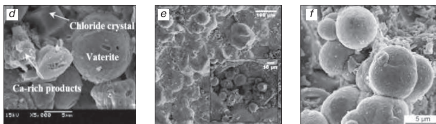
Рис. 9. Морфология кристаллических образований ватерита, сформированных под действием различных бактерий (слева направо): а – Sporosarcina pasteurii [6]; б – Bacillus subtilis [27]; с – Bacillus pasteurii [66]; д – Bacillus sphaericus [60]; е – Bacillus sphaericus [69]; ф – Myxococcus xanthus [68]
