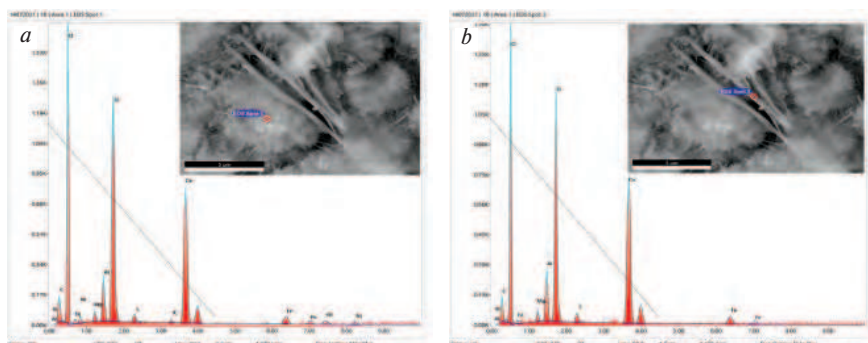
Рис. 5. Рентгеновский микроанализ новообразований с центрами кристаллизации, включающими никель/углеродный нанокompозит (а), и вторичных кристаллогидратов на основе гидросиликатов кальция в цементной матрице с никель/углеродными нанокompозитами (б)
