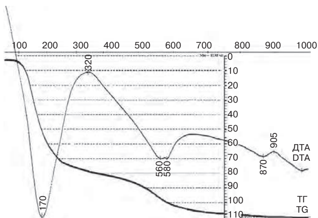
Рис. 3. Дериватограмма гипсокерамического состава, затворенного 11%-м раствором хлорида натрия
