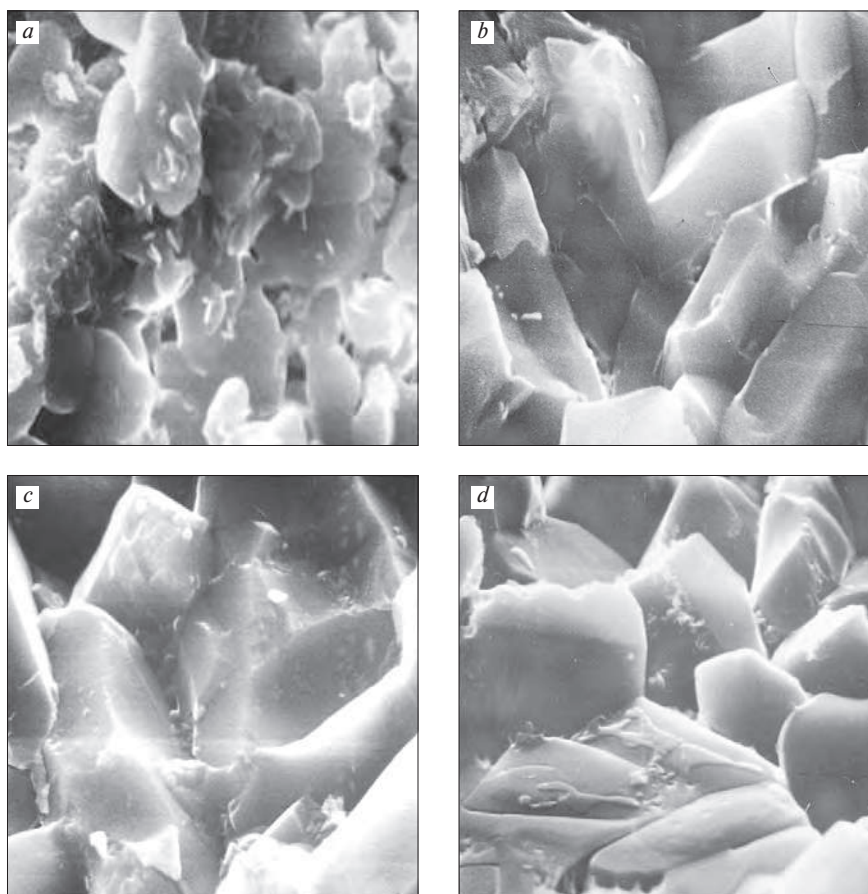
Рис. 6. Микроструктура гипсокерамических композиций при увеличении 3000×, приготовленных с концентрацией раствора хлорида натрия: а – 0%; б – 11%; с – 22%; д – 30%
