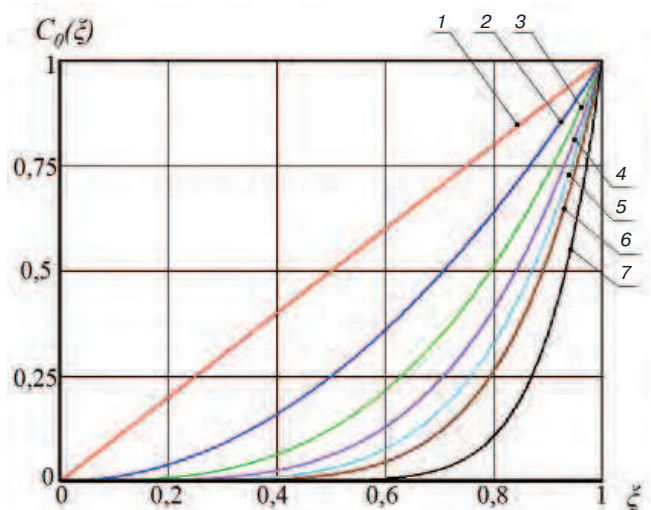
Рис. 3. Иллюстрация степенной зависимости вида \xi^n при различных показателях степени n : 1 – 1; 2 – 2; 3 – 3; 4 – 4; 5 – 5; 6 – 6; 7 – 10
