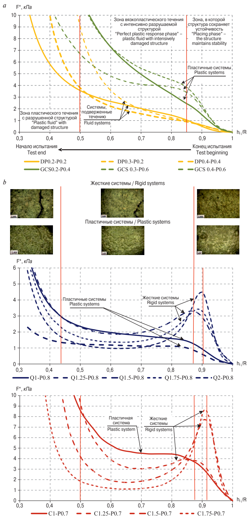
Рис. 1. Экспериментальные кривые F^* = f(h_i/R) для систем: а – «цемент – микронаполнитель – пластификатор – вода»; б – «цемент – мелкий заполнитель – пластификатор – вода» Fig. 1. Tested 3D-printable pastes F^* = f(h_i/R) curves for systems: а – «cement – filler – plasticizer – water»; б – «cement – aggregate – plasticizer – water»
